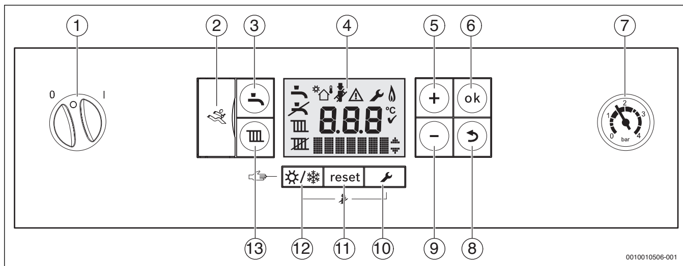
Fig. 1 Tableau de commande avec cache ouvert
